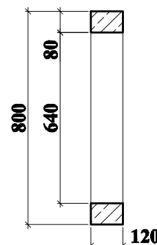
PRZEKRÓJ A-A
